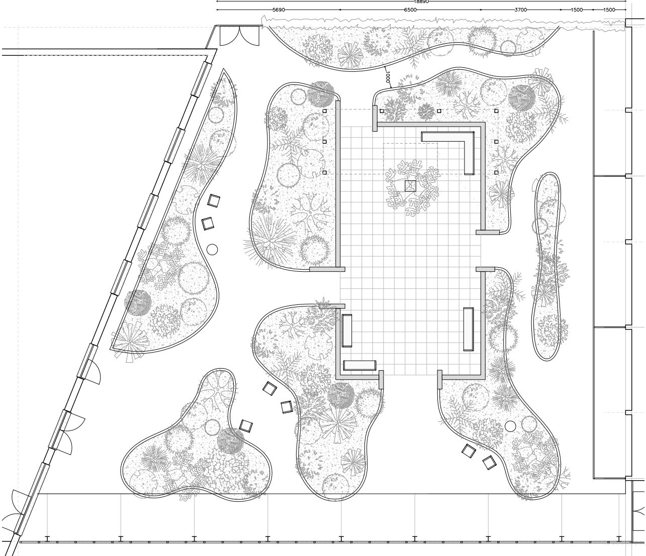
Technische Plattegrond
